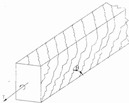
شکل ۱۲-۱۰- ترکهای پیچشی
