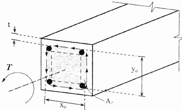
شکل ۸-۱۲ - لوله جدار نازک تحت اثر پیچش
