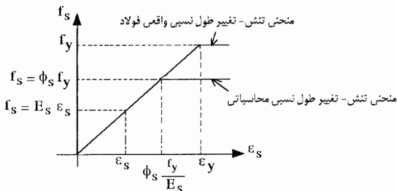
شکل ۱-۱۱ منحنی تنش - تغییر طول نسبی واقعی و محاسباتی فولاد
