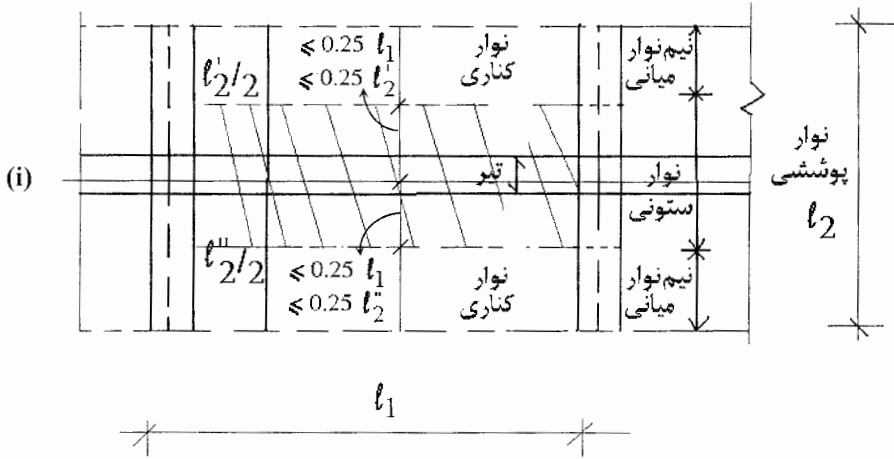
شکل ۱۵-۲ نوار ستونی و نیم نوارهای میانی
