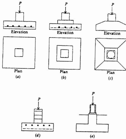
شکل ۱۷-۱ الف- انواع شالوده منفرد
