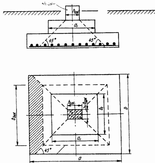
شکل ۱۷-۵ نمونه محل پله‌ها در شالوده پلکانی
