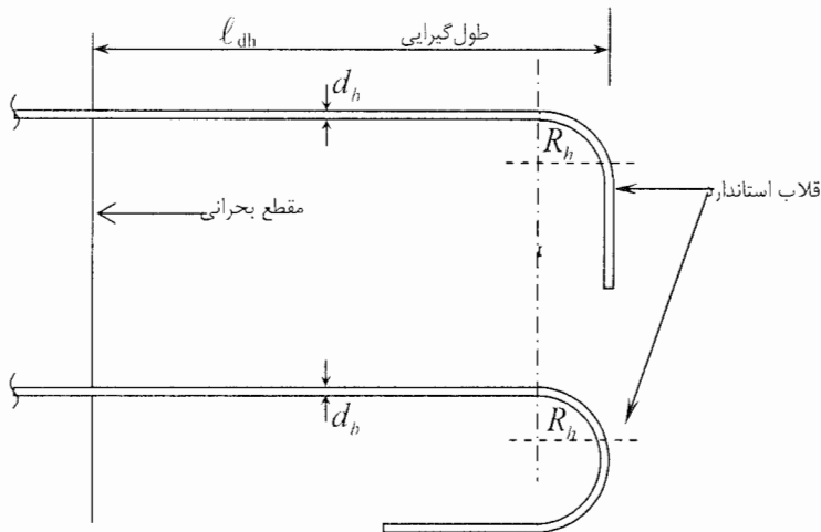
شکل ۱۸-۳ طول گیرایی میلگرد قلاب‌دار
