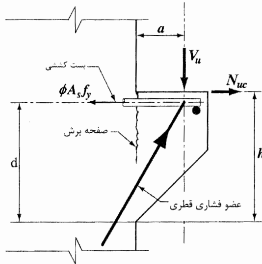
شکل ۱۲-۱۹- عملکرد سازه‌ای دستکها
