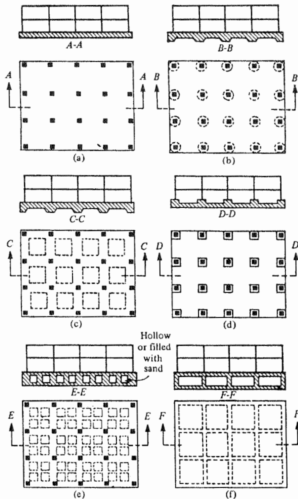
شکل ۱۷-۱ پ - انواع شالوده گسترده
