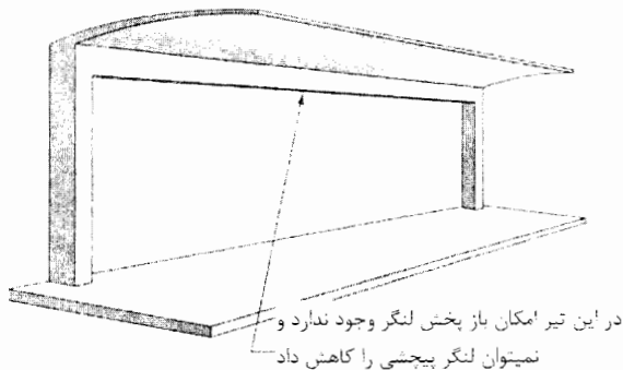
شکل ۱۲-۱۴- لنگر پیچشی غیرقابل کاهش
