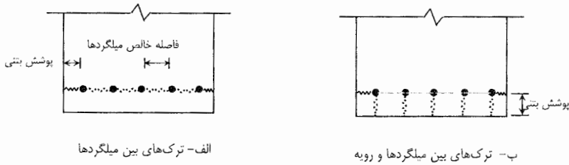
شکل ۱۸-۱ انهدام موضعی پیوستگی
