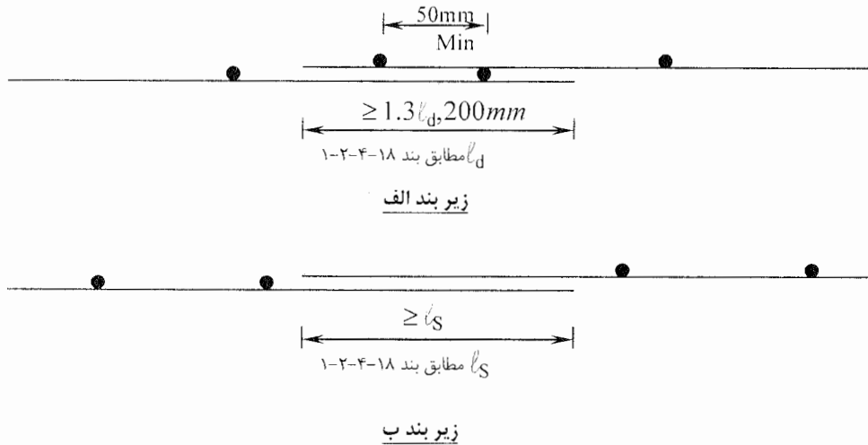
شکل ۱۸-۴ وصله پوششی در شبکه‌های جوش شده آجدار
