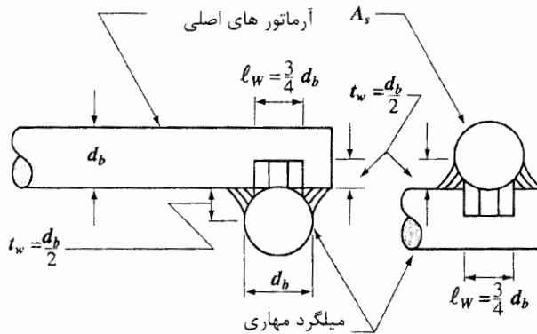
شکل ۱۲-۲۱- جزئیات جوش مهارها
