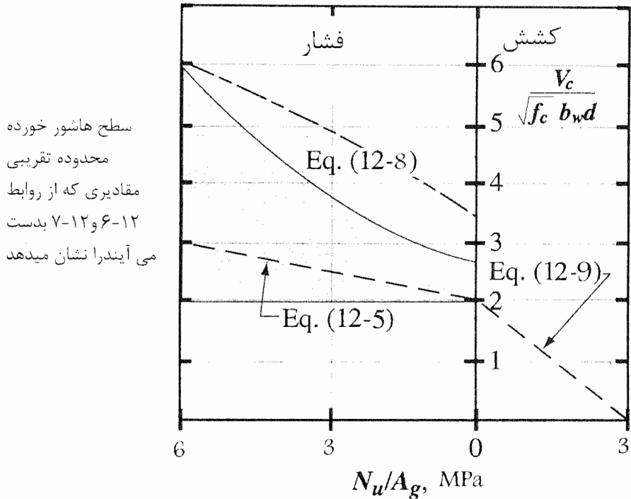
شکل ۱۲-۱ مقایسه روابط مقاومت برشی در اعضای تحت بار محوری
