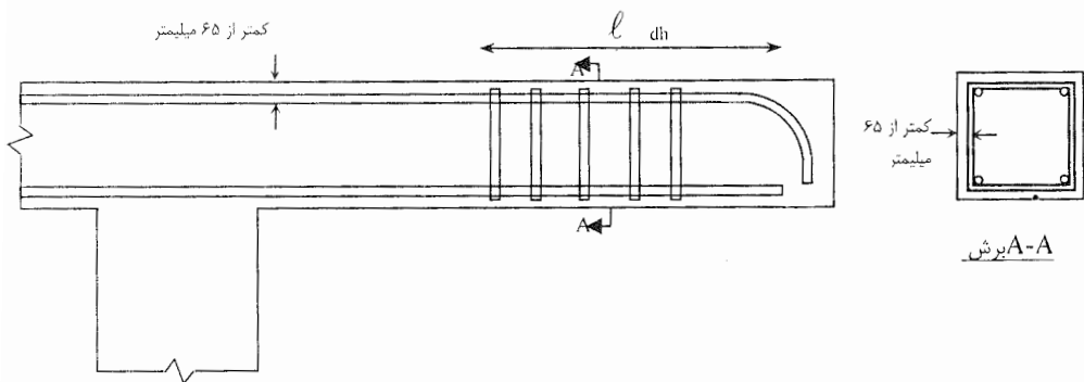
شکل ۱۸-۴ محصور کردن بتن در ناحیه قلاب
