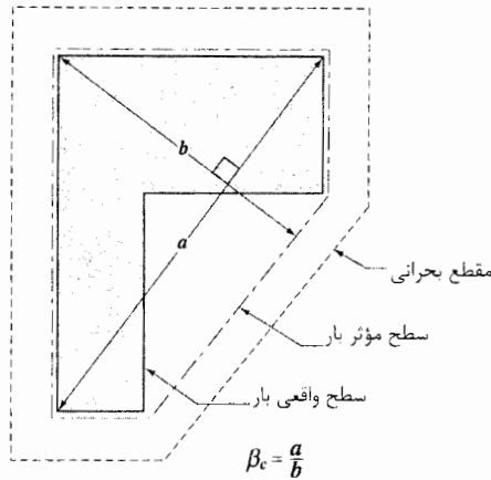
شکل ۱۲-۲۲- مفادیر \beta_c برای سطوح بارگیر غیرمستطیلی
