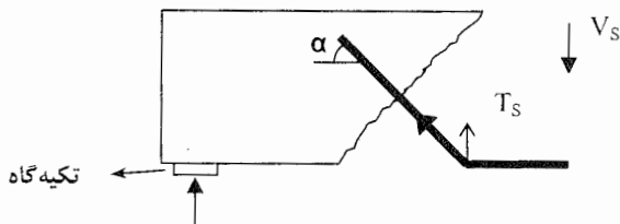
شکل ۱۲-۲: اثر آرماتورهای خم شده در برش
