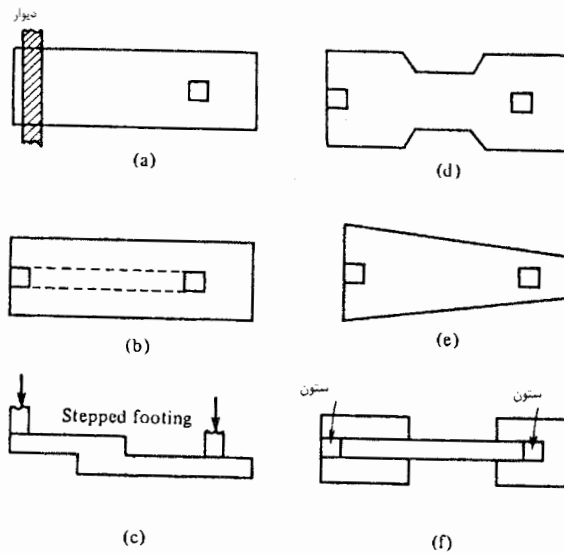
شکل ۱۷-۱ ب- انواع شالوده نواری
