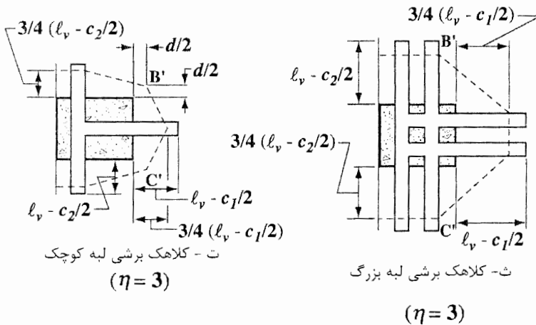
شکل ۱۲-۲۶- موقعیت مقطع بحرانی
