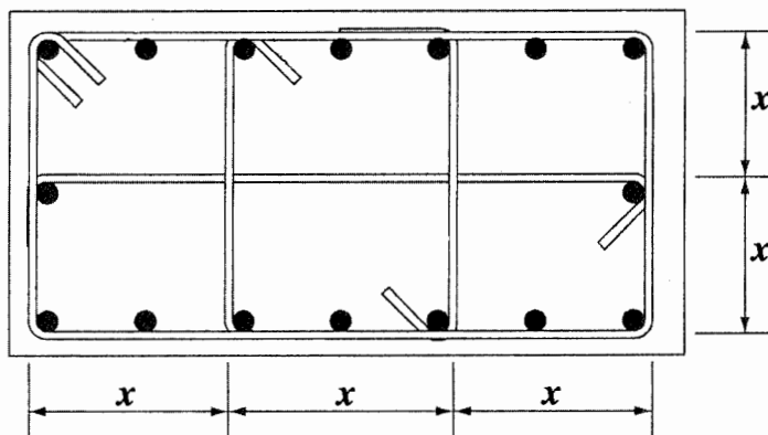
شکل ۳-۲۰ نمونه‌ای از آرماتور عرضی در ستونها
