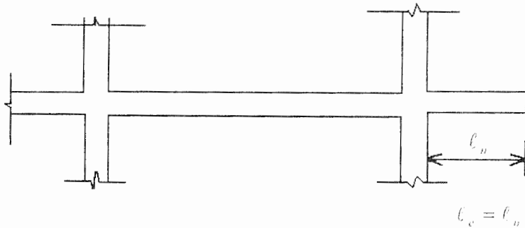
شکل ۱۰-۳-۳-پ - طول دهانه موثر در اعضای طره‌ای
