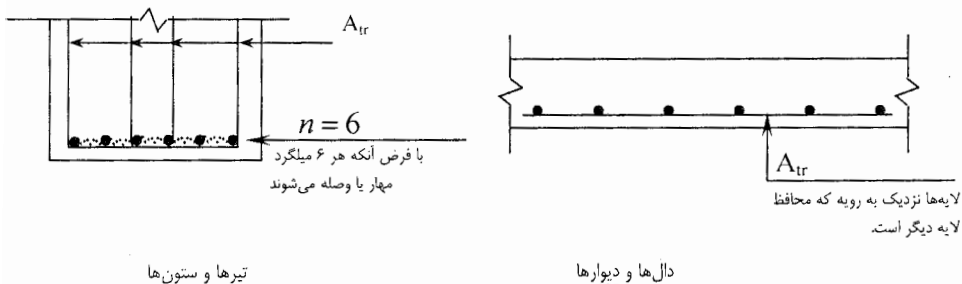
شکل ۱۸-۲ ضریب A_{tr}
