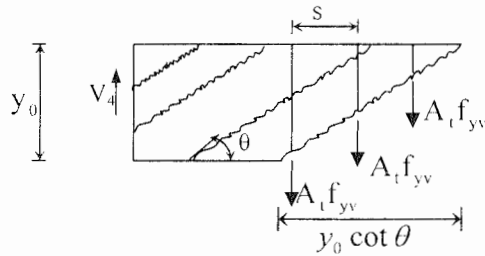
شکل ۱۲-۱۲- کشش قائم در خاموتها
