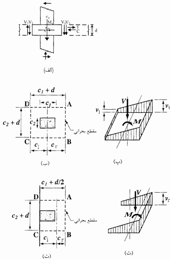
شکل ۱۲-۲۹- انتقال لنگر از دال به ستون
