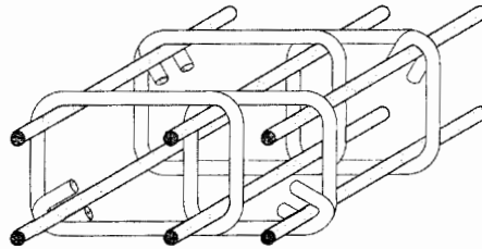
شکل ۱۲-۲۳- خاموت دالها
