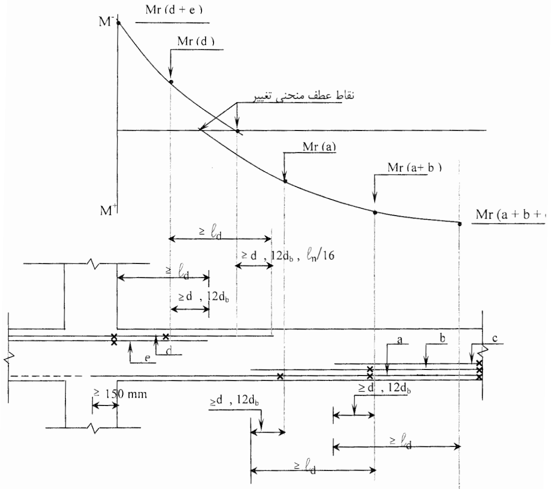
شکل ۱۸-۶ ضوابط مربوط به قطع میلگردها
