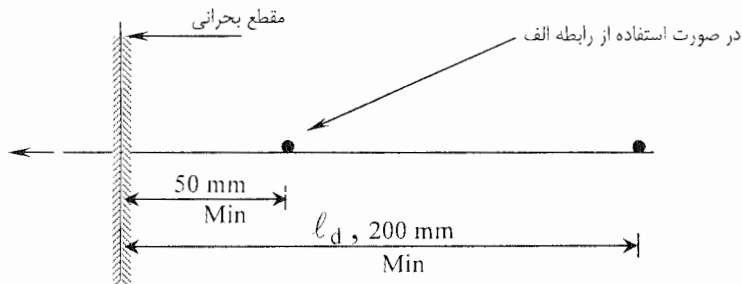
شکل ۱۸-۴ مهار شبکه‌های آجدار
