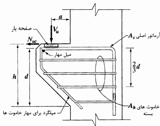
شکل ۱۲-۲۰- جزئیات دستکها
