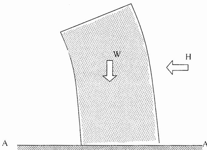
شکل ۲۰-۴ بارهای وارده به یک دیوار
