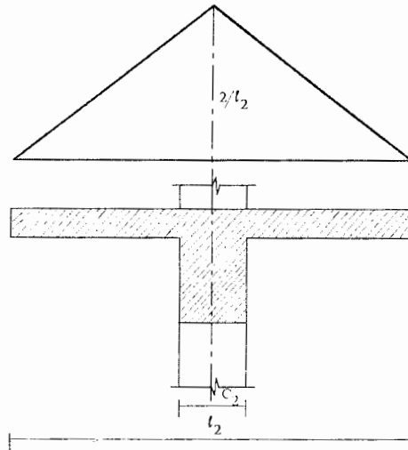
شکل ۱۵-۶ چشمه دال
