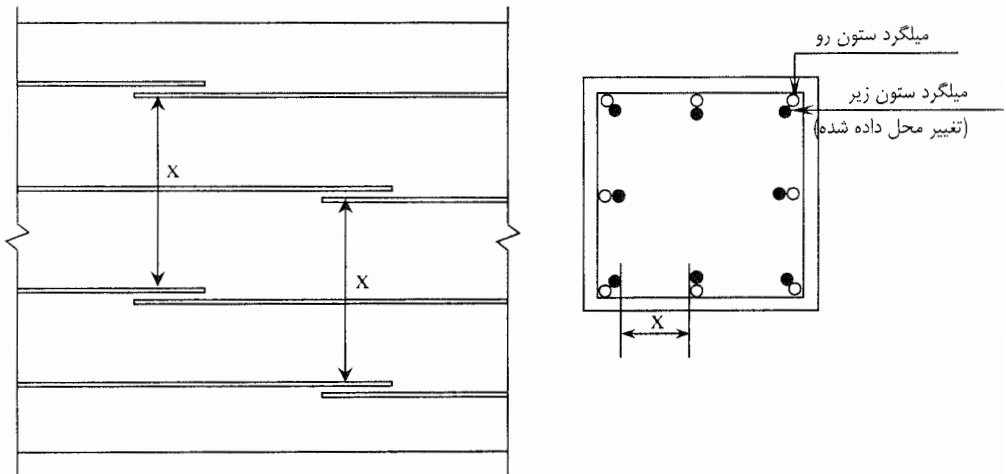
شکل ۱۸-۱۳ فاصله میلگردهای مشابه از یکدیگر
