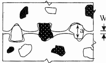
شکل ۱۲-۱۷- قفل و بست مصالح سنگی در محل ترک
