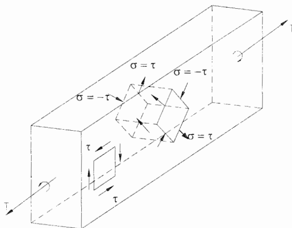
شکل ۱۲-۹- تنش های ایجاد شده در اثر پیچش
