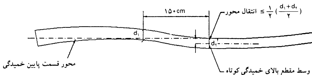
شکل ۱۳-۵ خمیدگی کوتاه تیر، حالت سوم.
