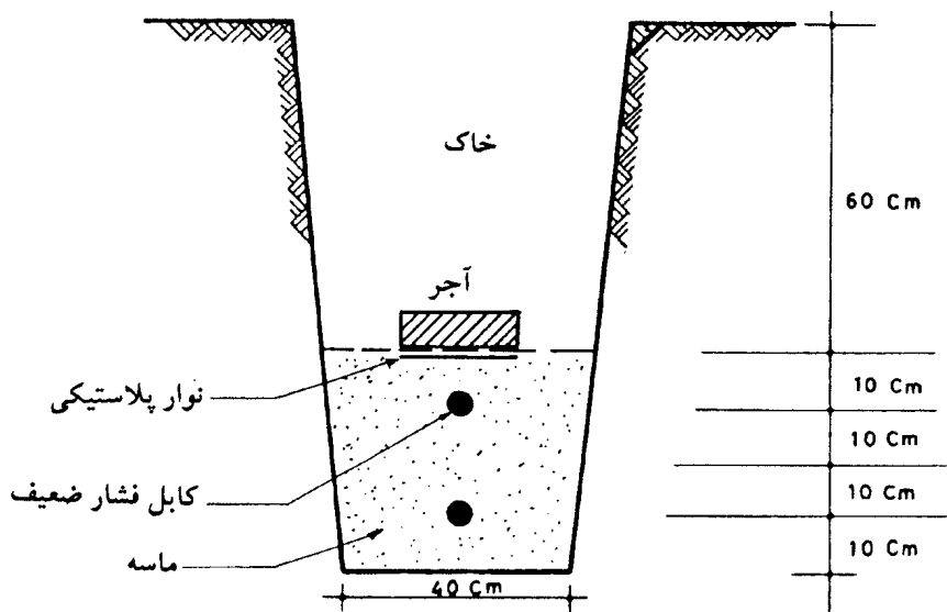
جزئیات کانال خاکی تیپ برای نصب کابل فشار ضعیف در دو ردیف افقی
