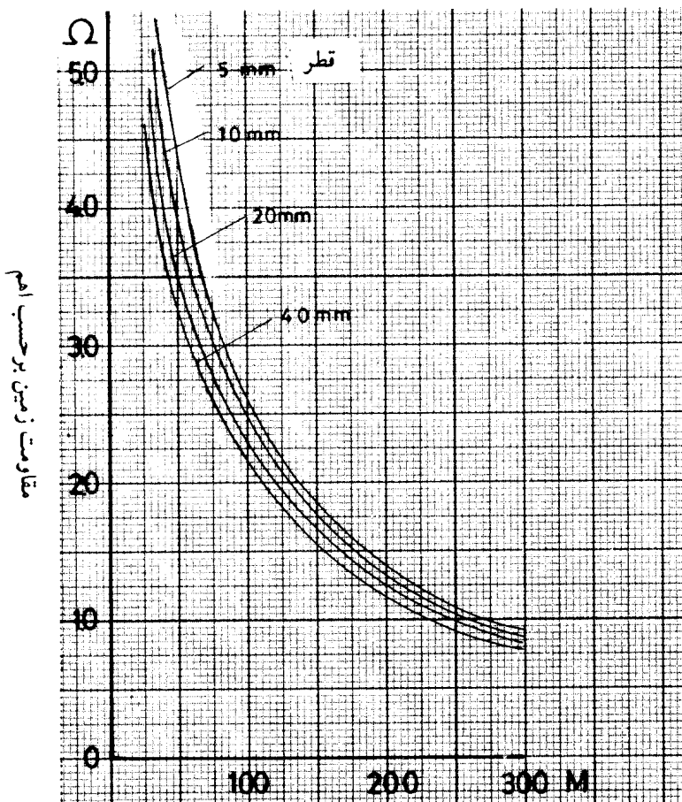
طول الکترود بر حسب متر
