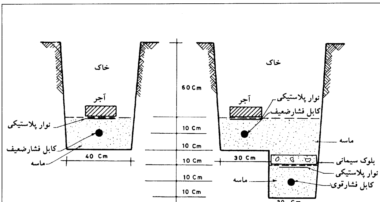
جزئیات کانال خاکی تیپ برای نصب کابل فشار ضعیف در یک ردیف افقی
