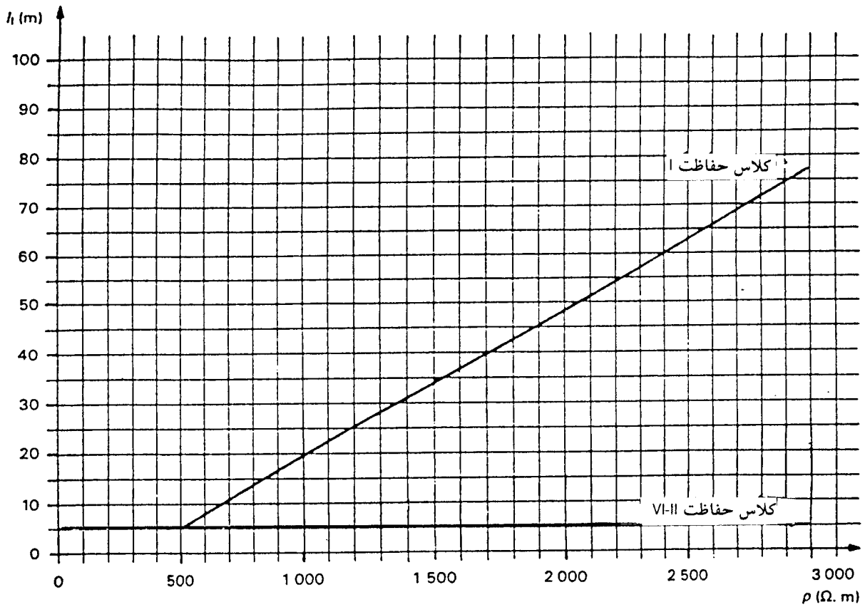
شکل ۱۴-۲ حداقل طول الکترودهای پایانه زمینی برحسب کلاس حفاظت و میزان مقاومت زمین برابر استاندارد IEC 1024-1.
