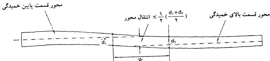
شکل ۱۳-۳ خمیدگی کوتاه تیر، حالت اول.
