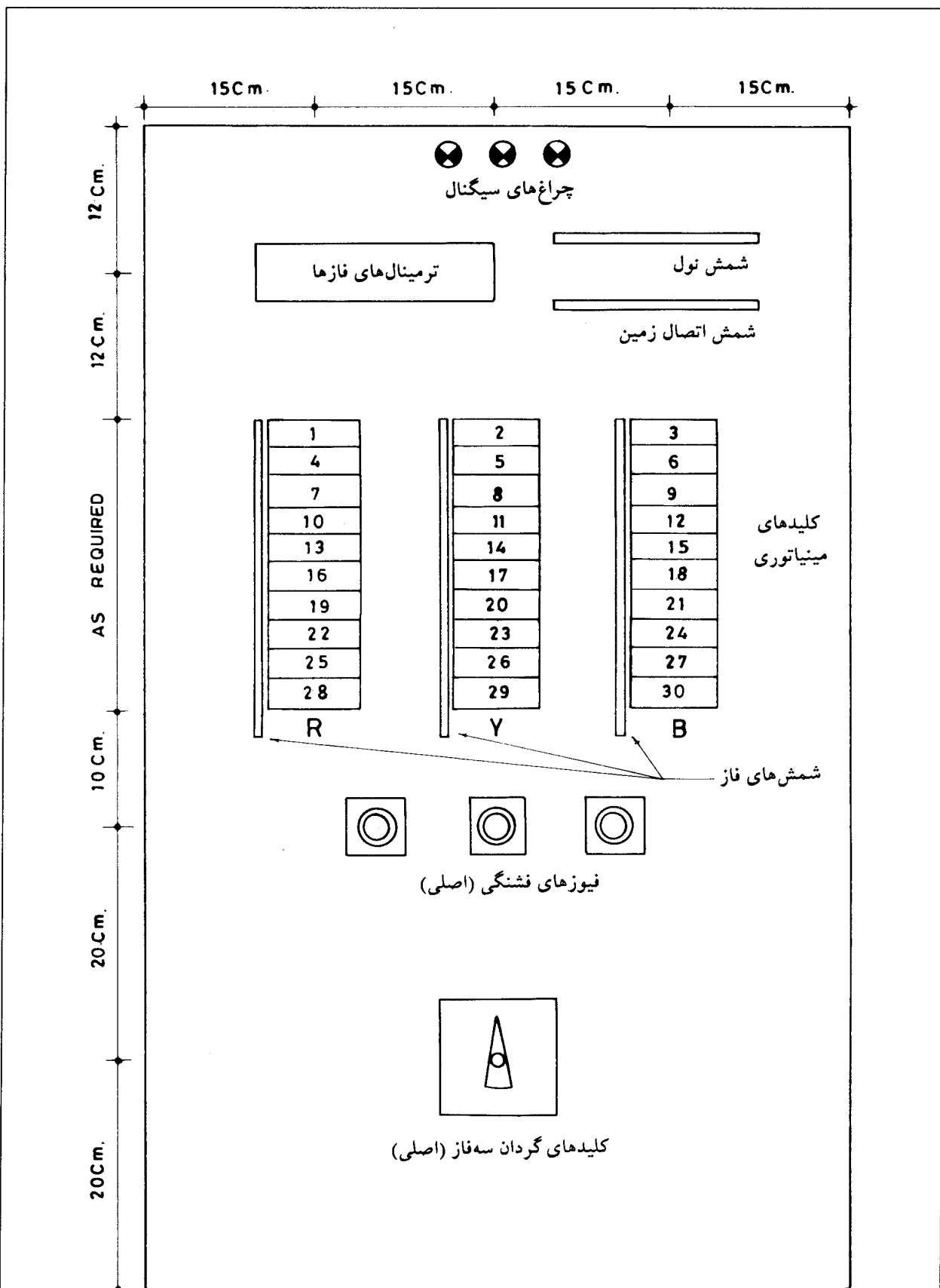
سیستم استقرار وسایل با حداقل فواصل در داخل تابلوی فرعی توزیع برق - نوع سه فاز.
