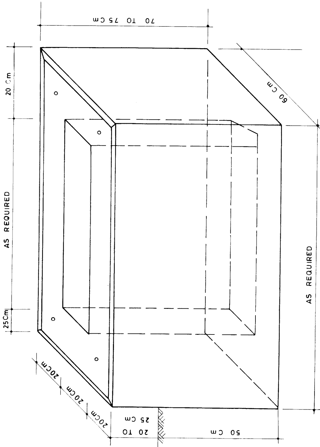
شکل ۵-۲۰ سکوی مخصوص نصب تابلوهای توزیع نیروی برق قابل نصب در فضای باز.
