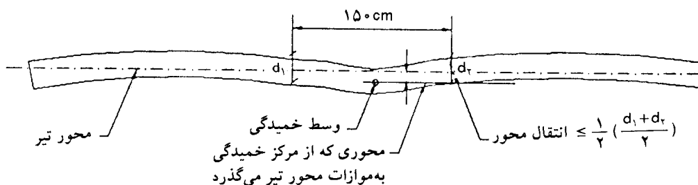
شکل ۱۳-۴ خمیدگی کوتاه تیر، حالت دوم.
