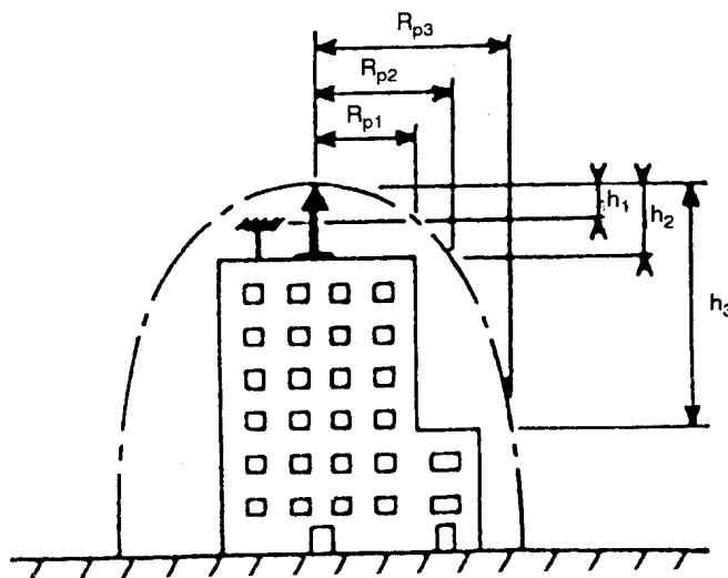
شکل ۱۴-۷ محدوده و شعاعهای حفاظت برقگیر الکترونیک.
