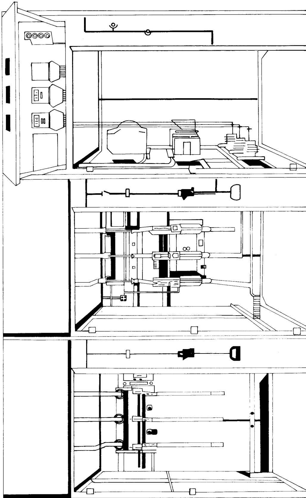
شکل ۱-۶ تابلوی فشار متوسط نوع قابل دسترسی از جلو.
