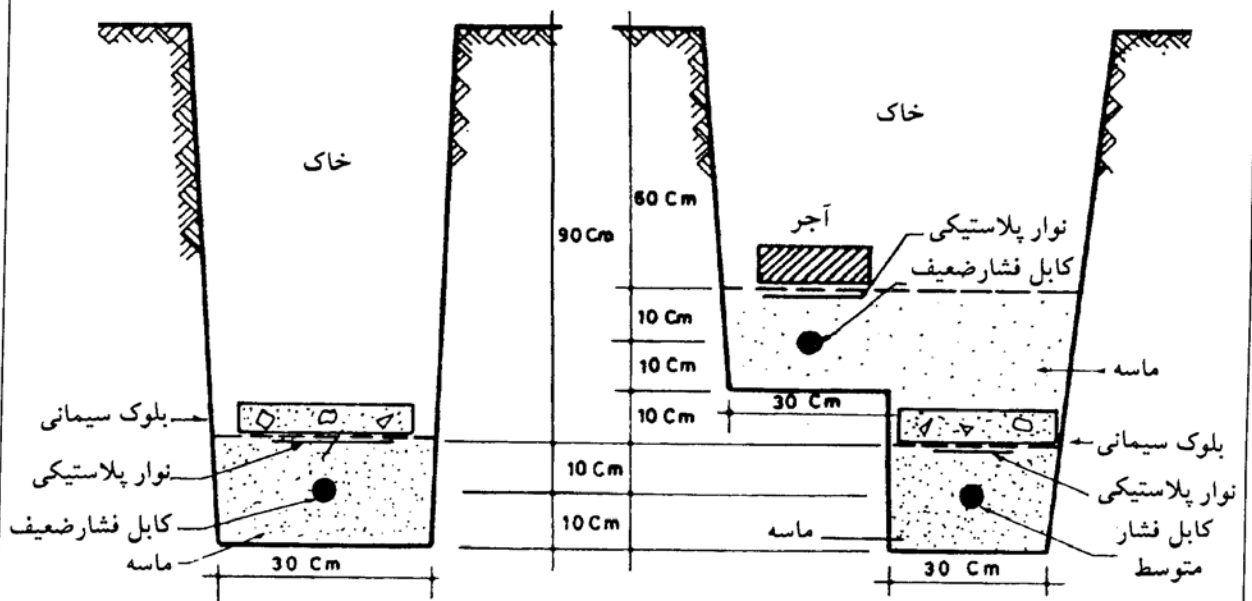
جزئیات کانال خاکی تیپ برای نصب کابل فشار متوسط در یک ردیف افقی
