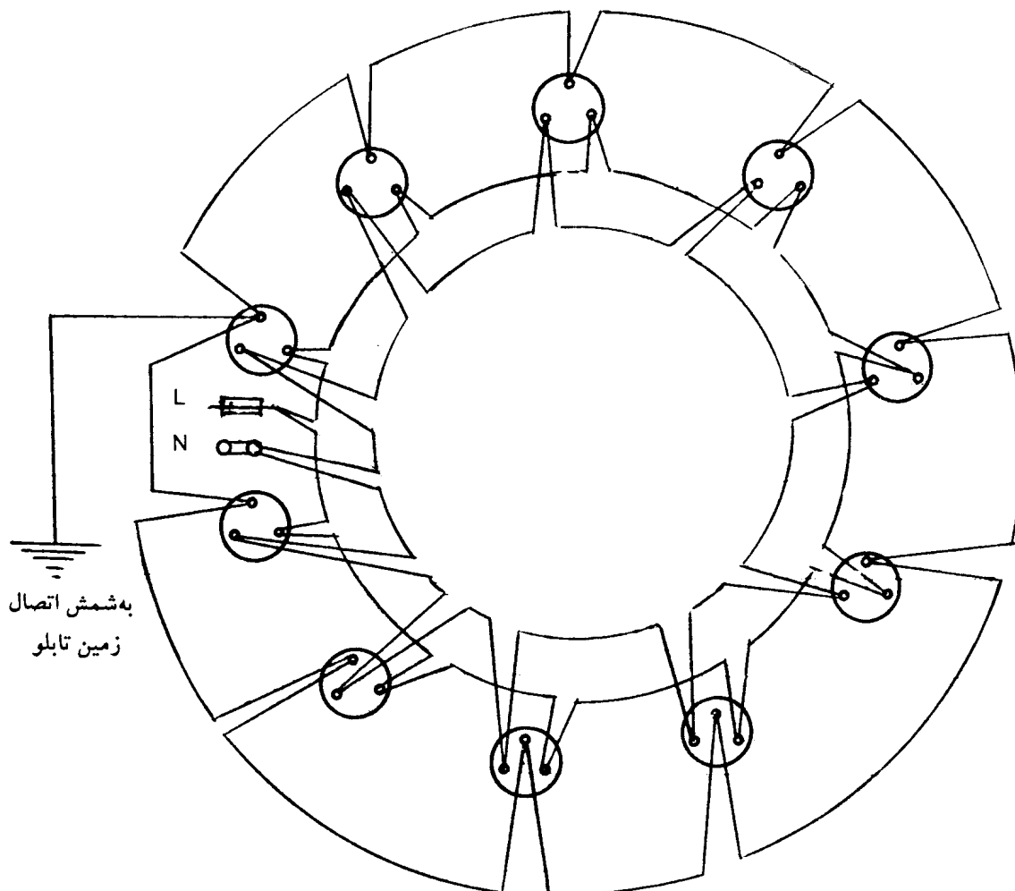
شکل ۲-۳ سیستم سیمکشی حلقوی مدار پریزها.
