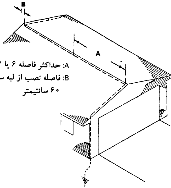
(الف) فواصل نصب بر روی خط الرأس سقفهای شیبدار
