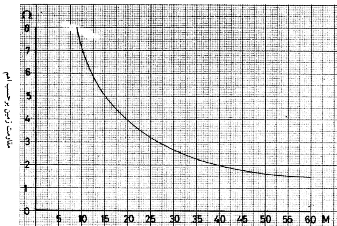
طول هر الکترود بر حسب متر
