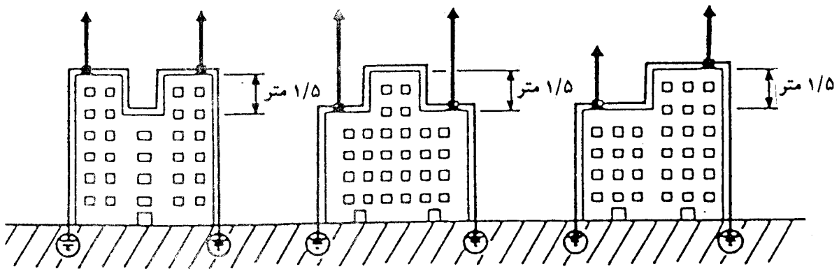
(الف) اتصال پایانه‌های هوایی الکترونیک به یکدیگر با اختلاف سطح حداکثر ۱/۵ متر
