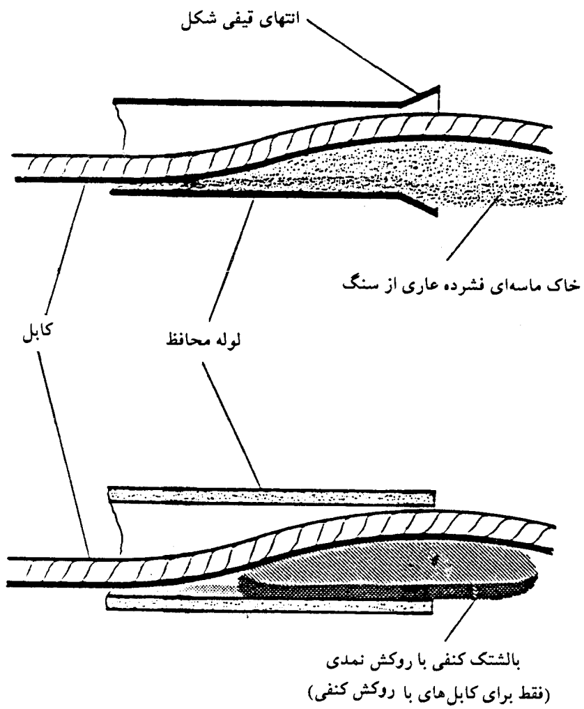
شکل ۸-۲ حفاظت کابل در مدخل ورودی لوله
