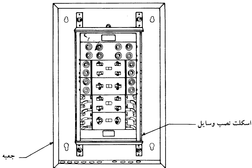
جعبه و اسکلت تابلوی دیواری (الف)
