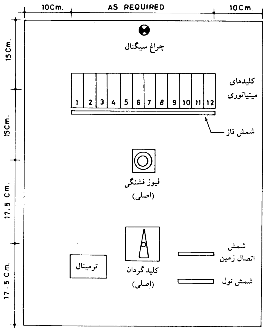
سیستم استقرار وسایل با حداقل فواصل در داخل تابلوی فرعی توزیع برق - نوع یک فاز.
