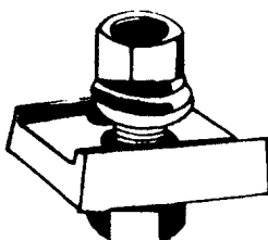
۱۲ - بست تسمه به فلز (ورق و یا پروفیل)
