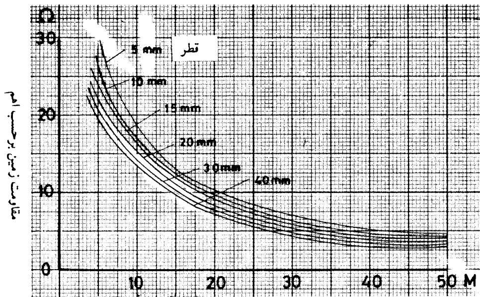
طول الکترود بر حسب متر
