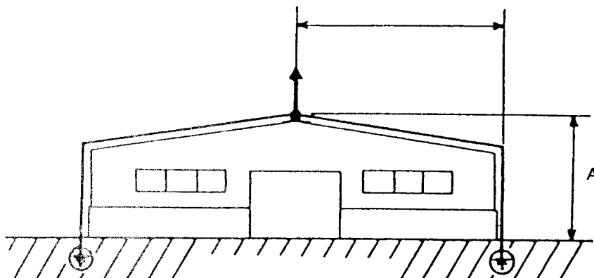
(پ) A < 28 متر یا B > A : دو هادی نزولی
