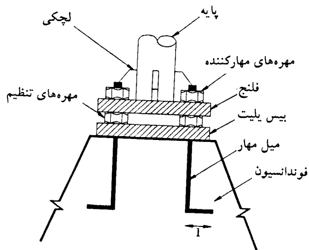
جزئیات نصب پایه بر روی فونداسیون بتنی پیش ساخته شکل ۸-۱۳
