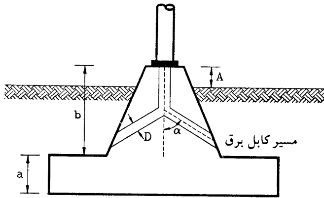
نمای نمونه فونداسیون بتنی پیش ساخته شکل ۷-۱۳
