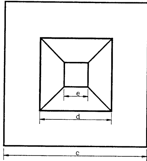
پلان نمونه فونداسیون بتنی پیش ساخته شکل ۶-۱۳
