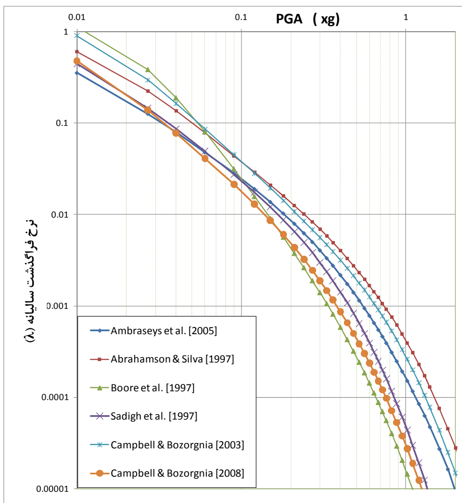
شکل ۳-۴- تحلیل حساسیت منحنی‌های خطر به روابط کاهندگی در یک ساختمان فرضی
