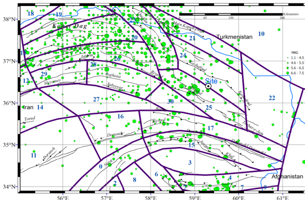
شکل ۳-۱- انتخاب پهنه‌های لرزه‌ای و چشمه‌های خطی و سطحی (برگرفته از گزارش تحلیل خطر زلزله منطقه‌ای در خراسان رضوی. ذوالفقاری، آشتیانی، مختاری، ۱۳۹۱)
