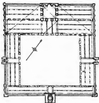
۸۳ - قاهره - طرح دوبار مسازشده مسجد سلطان بیبرس (۱۲۶۹ - ۱۲۶۷) .
