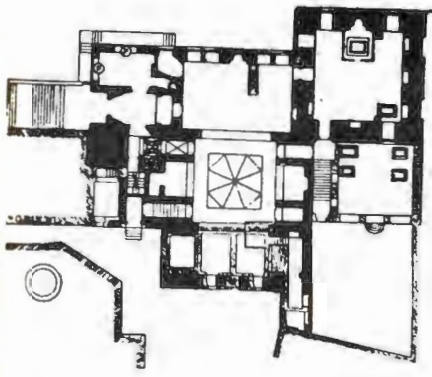
۹۱ - قاهره - طرح مدرسه و مقبره سلطان قائدیک.
