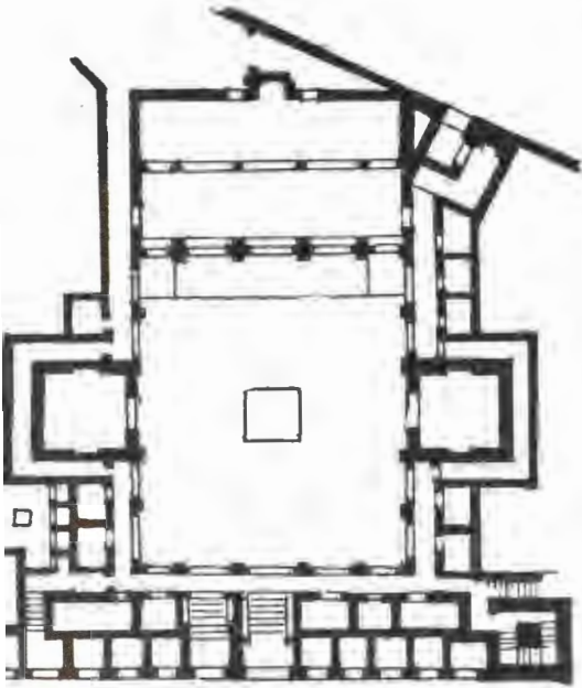
۶۳ - فاس (مراکش) - طرح بنای مدرسه «بوعنانیا» .. (۱۳۵۰-۱۳۵۵)
