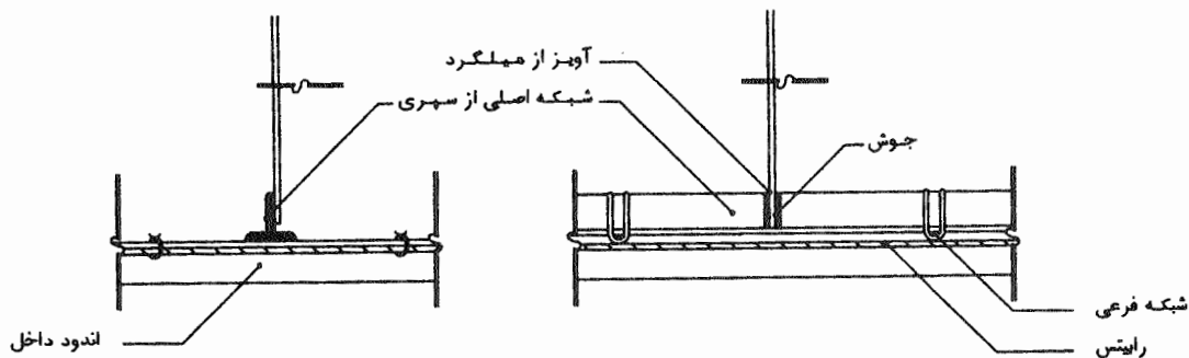
مقطع B-B
