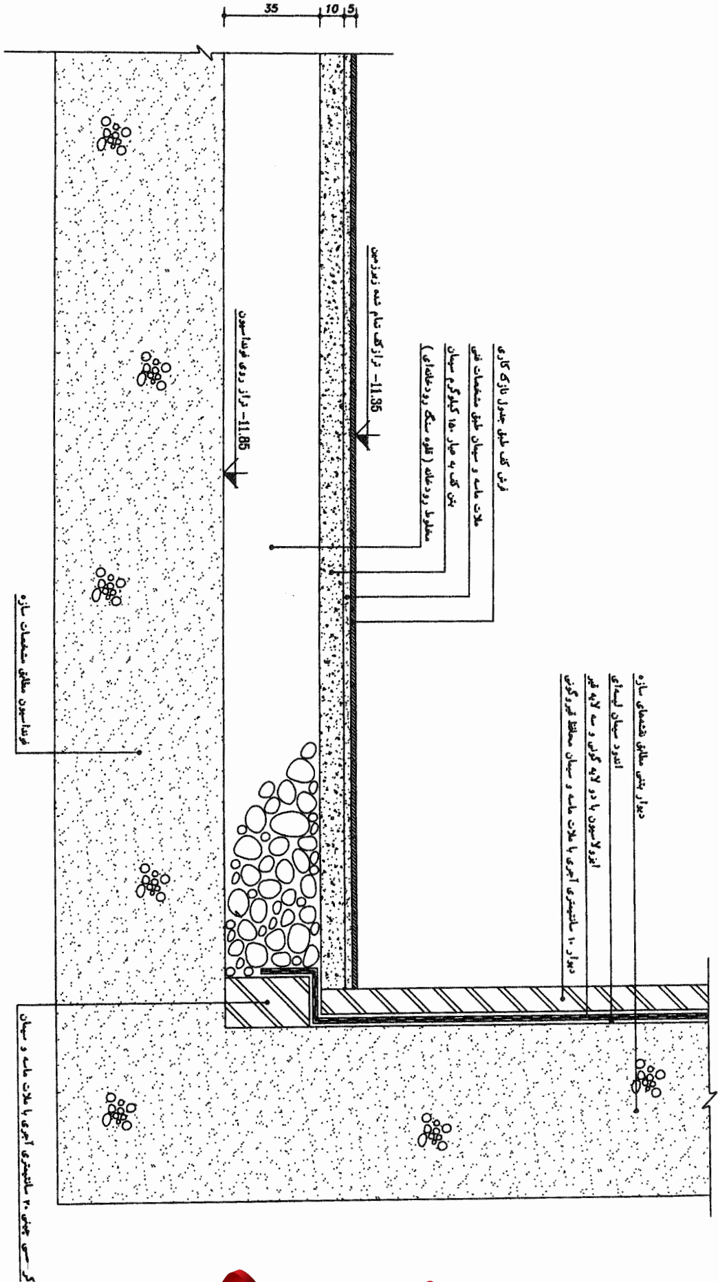
جزئیات ایزولاسیون دیوارهای خارجی در زیر زمین
