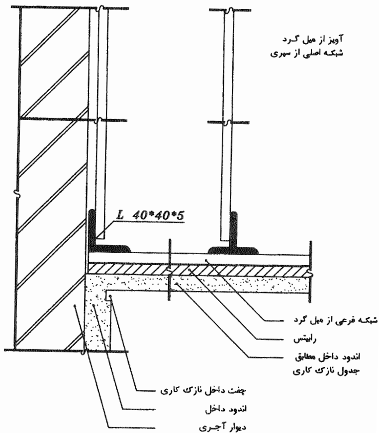
مقطع A-A
