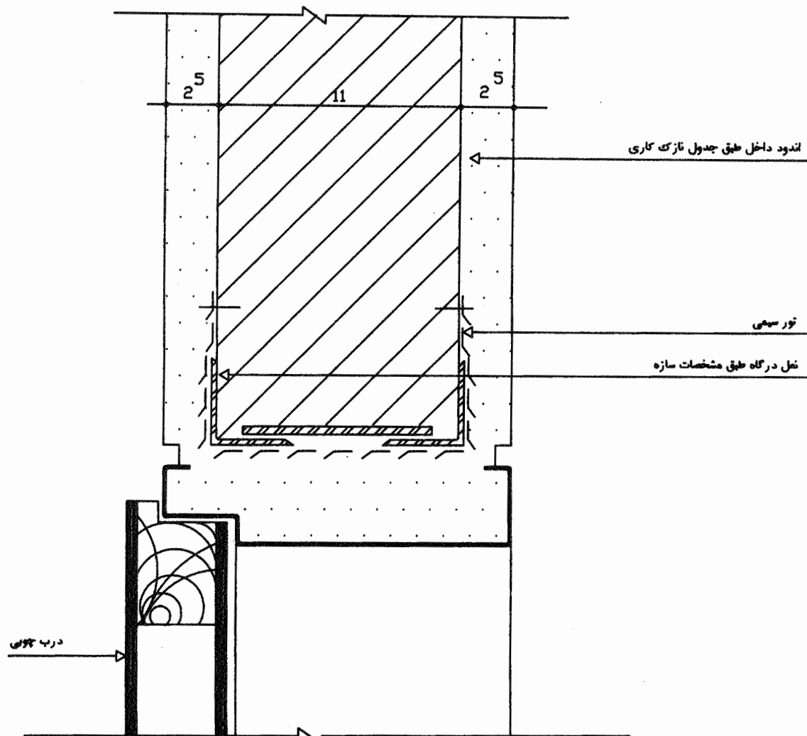
جزئیات اتصال دربهای چوبی
