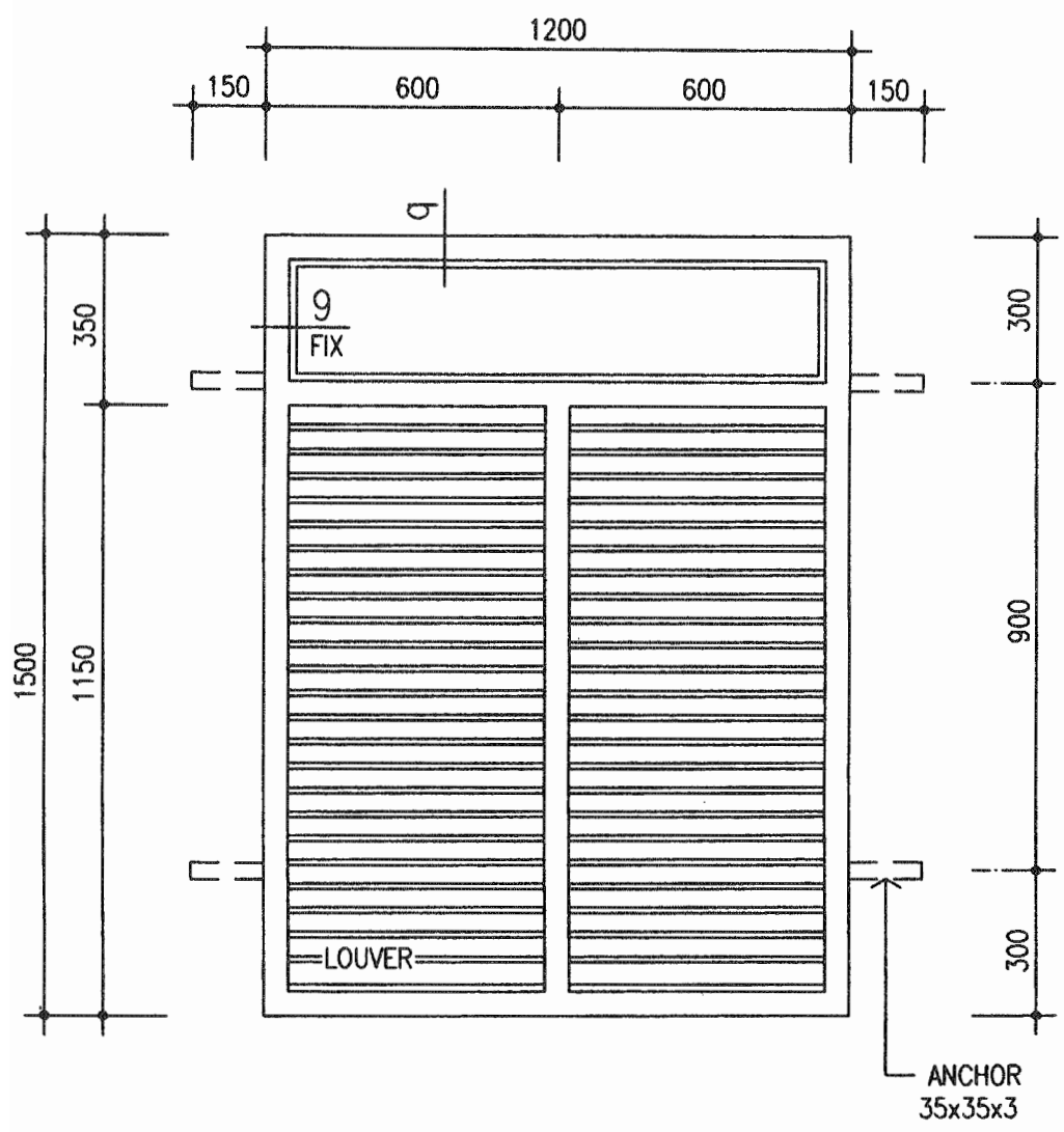
METAL LOUVER NO 4
