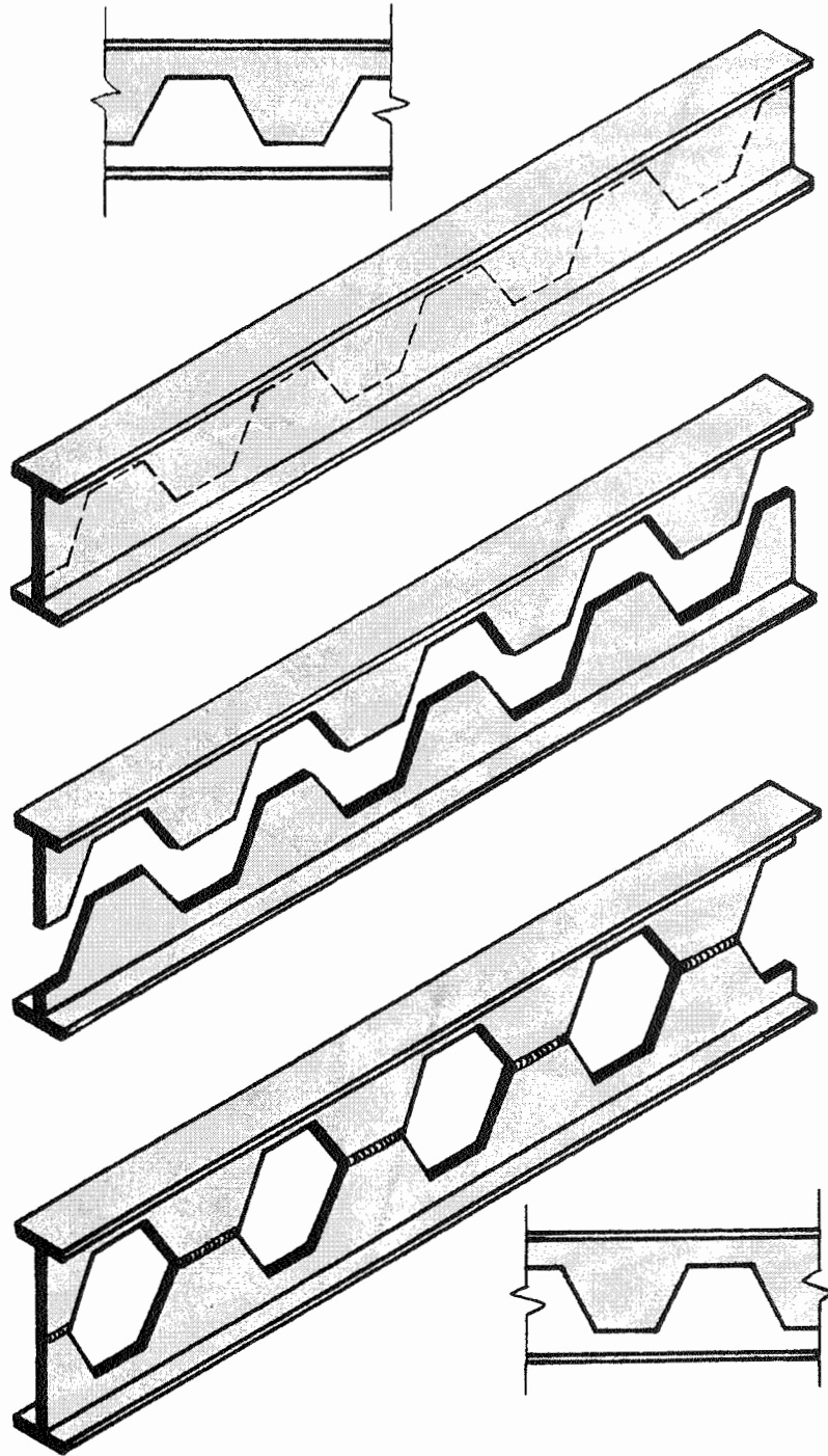
تبدیل تیر IPE به تیرلانه زنبوری
