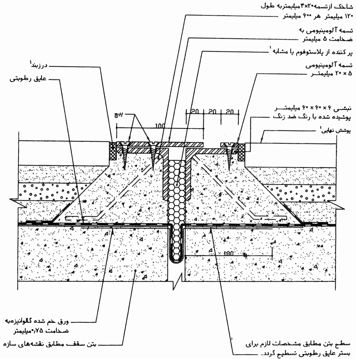
جزئیات درز انبساط در کف طبقات با عایق رطوبتی
