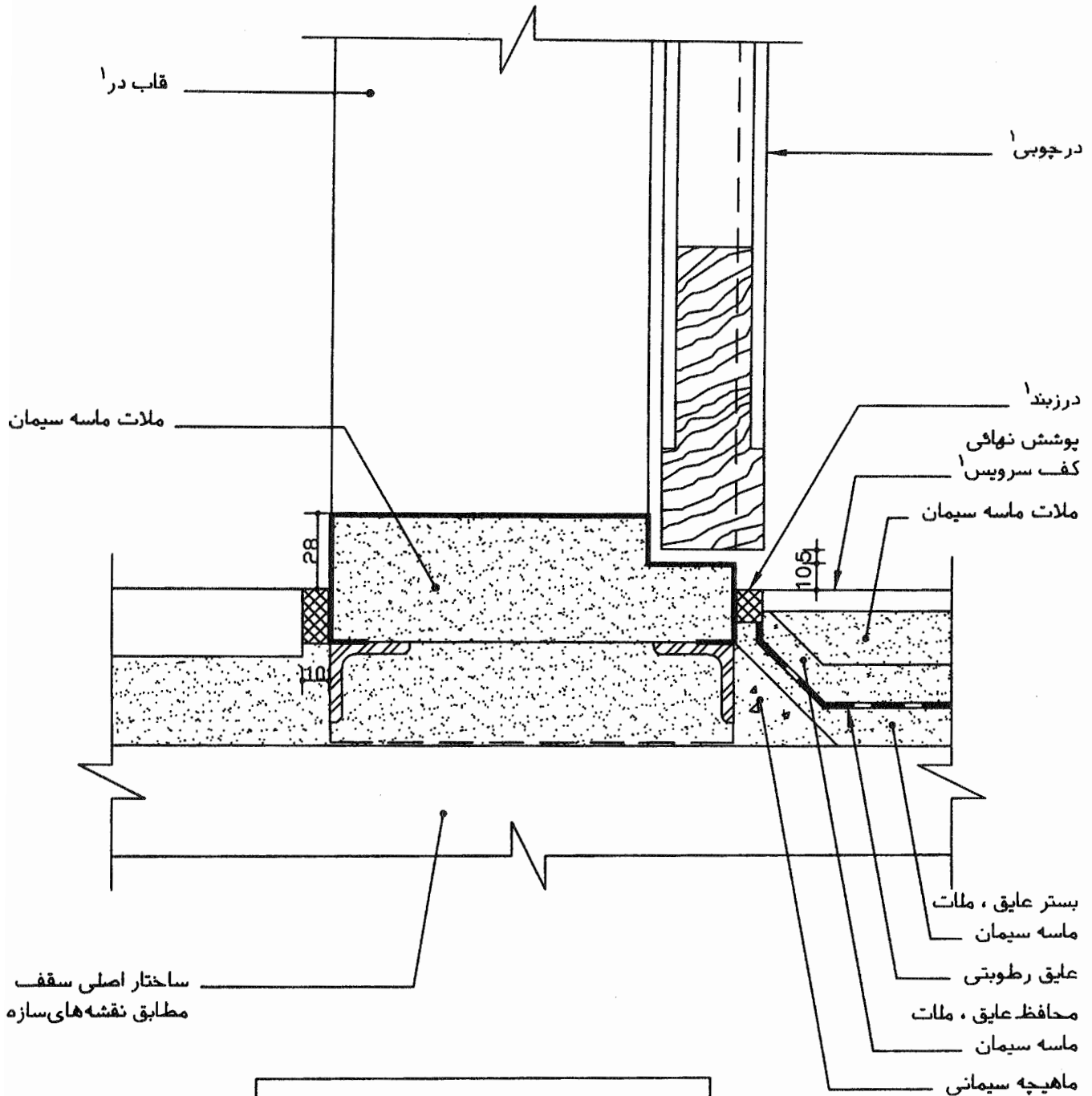
جزئیات اتصال آستانه در طبقات آستانه فلزی در کف سرویس یا آشپزخانه
