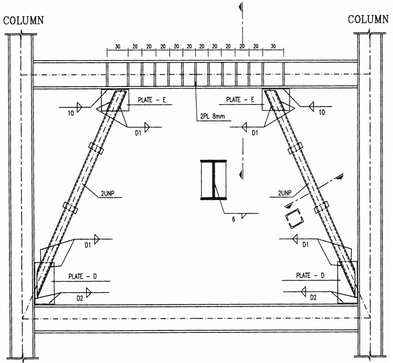
جزئیات بادبند پهای EBF
