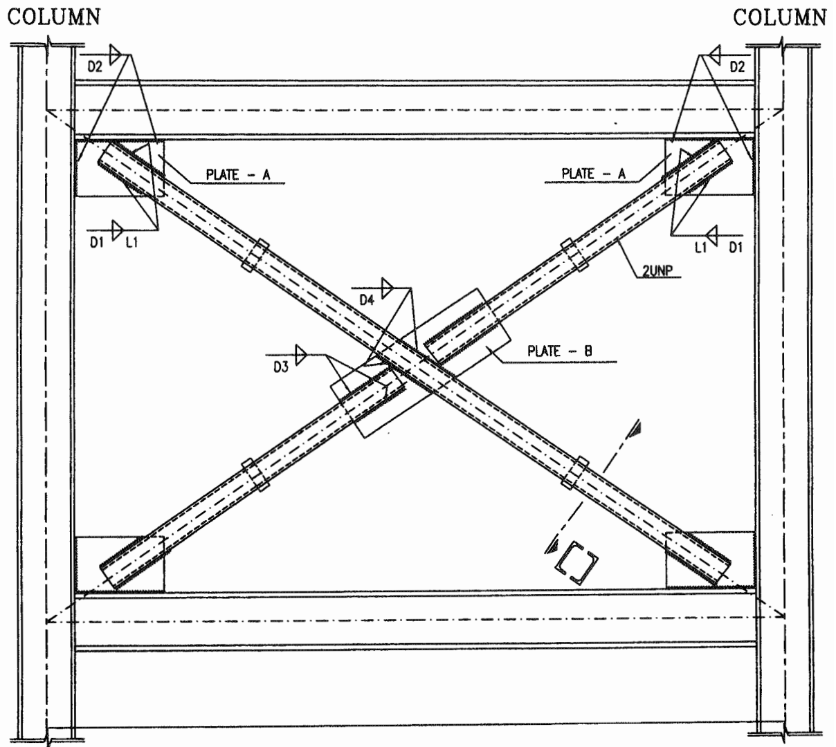
جزئیات بادبندی پای ضربدری
