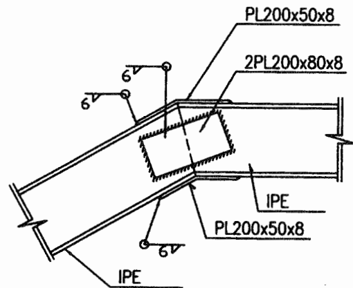
جزئیات تیر شمشیری راه پله
