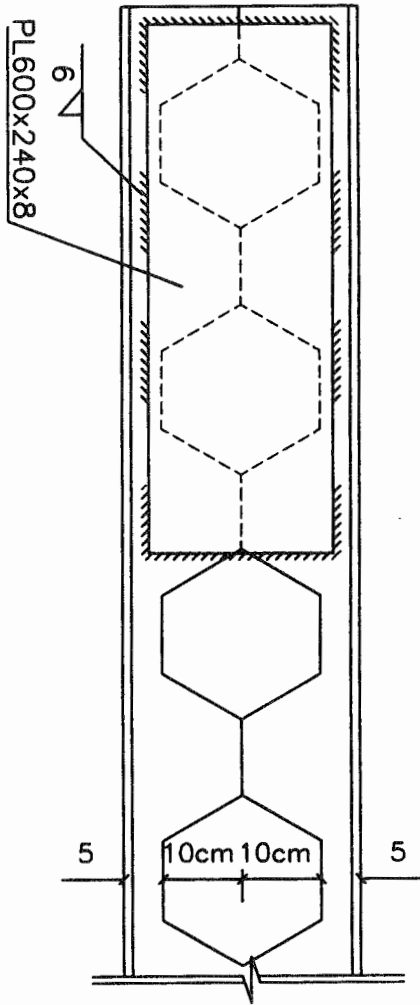
نحوه جوش ورق تقویتی جان در محل نایه گاه CPE200
