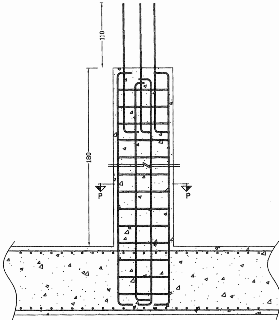
جزئیات پداستال
