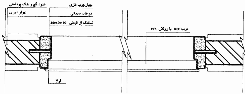
برش افقی از چهارچوب درب سرویسیها
