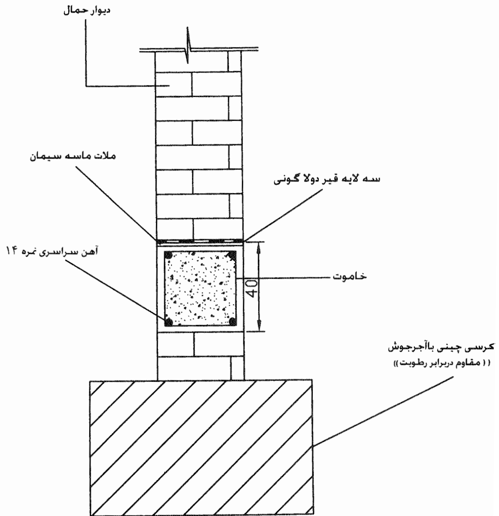
دیوار حمال با شناژ
