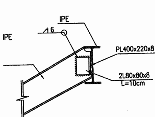
جزئیات تیر شمشیری راه پله
