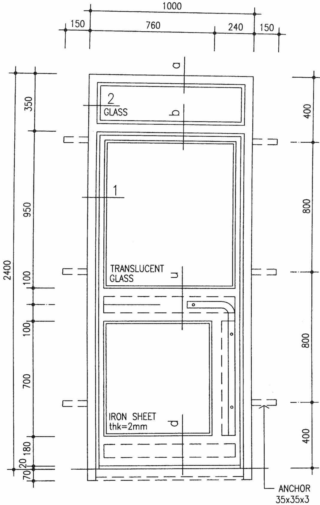
METAL DOOR NO 3
