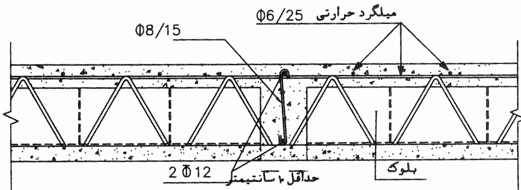
جزئیات اجرایی کلاف بتونی
