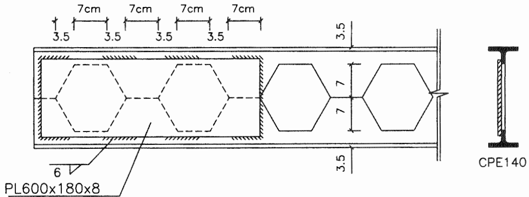
نخوه جوشی ورق تقویتی جان در محل تکیه گاه CPE140
