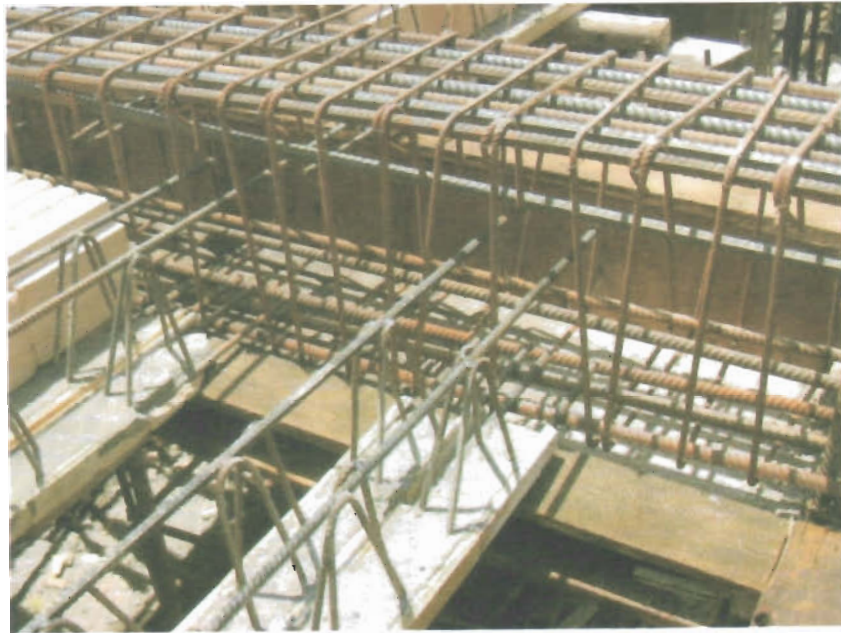
نحوه قرار گیری سر تیرچه ها به پوتر بتنی (به تیرچه دویل توجه فرمایید)
