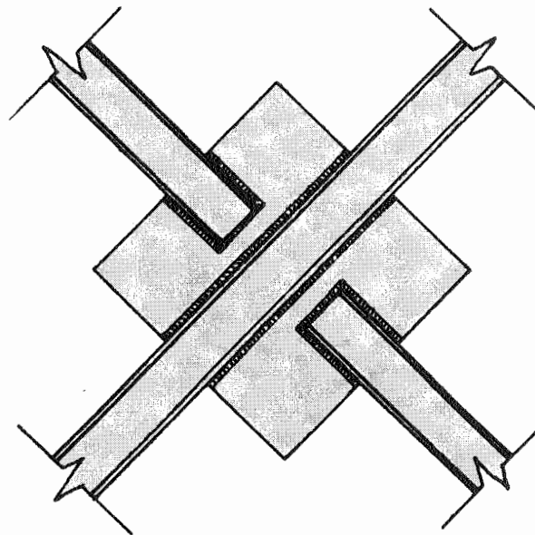
چگونگی اتصال ناودانی به ورق در بایندهای ضریبری
