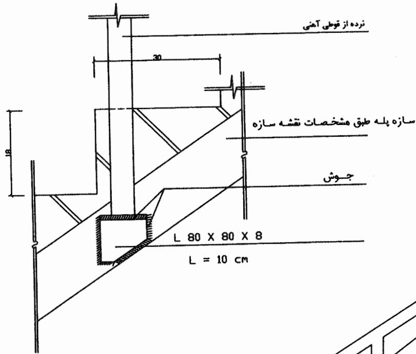
D-4 جزئیات اتصال نرده به پله
