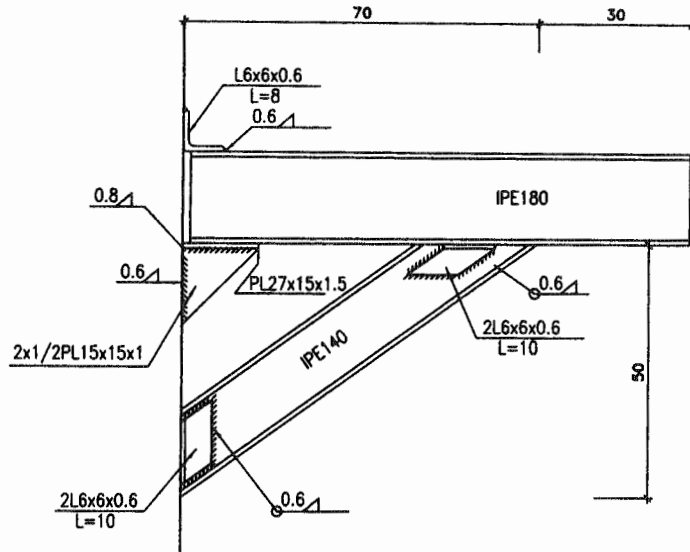
اتصال تیر کنسول با دستک فشاری
