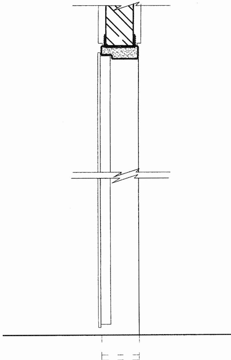
برش عمودی از چهارچوب درب سرویسیها
