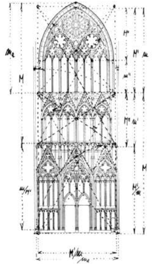
کلیسای سنت آتون ، مناکس تحلیل تناسبی بخشی از تقاطع گاه شمالی
